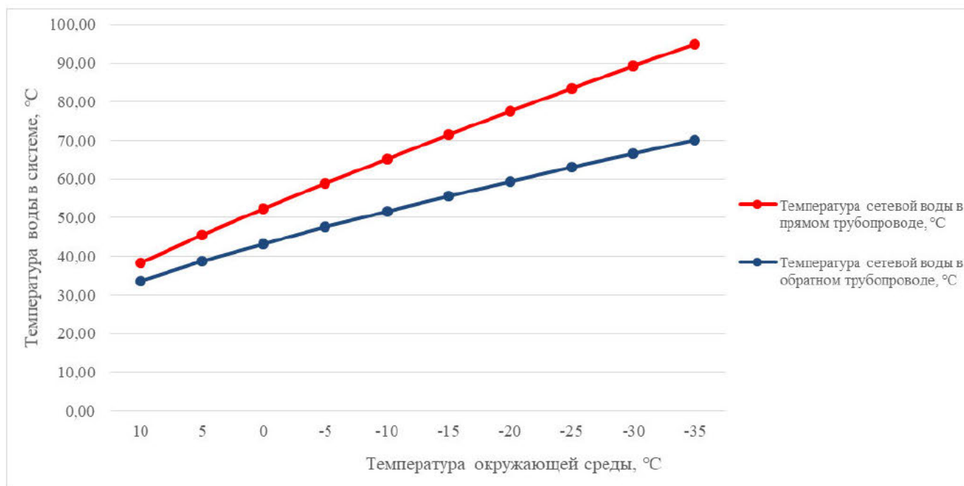
Рисунок 2.2 – График изменения температур теплоносителя котельной п. Новопокровка (температурный график 95/70^{\circ}\text{C} )
